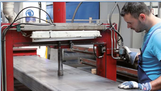
Option „Absetzvorrückung“: Bei Hebebühnen für die Fahrwerksvermessung wird jede Fahrfläche im Bereich der Drehteller- und Schiebepfattenauflagen nach dem Schweißen auf einer Vorrückung exakt eben gerichtet.
