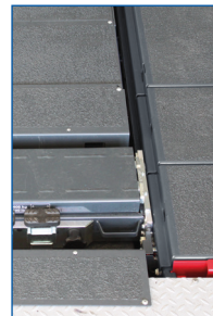
DUO CM im Streifenfundament (Ausstattung für Fahrwerksvermessung).
